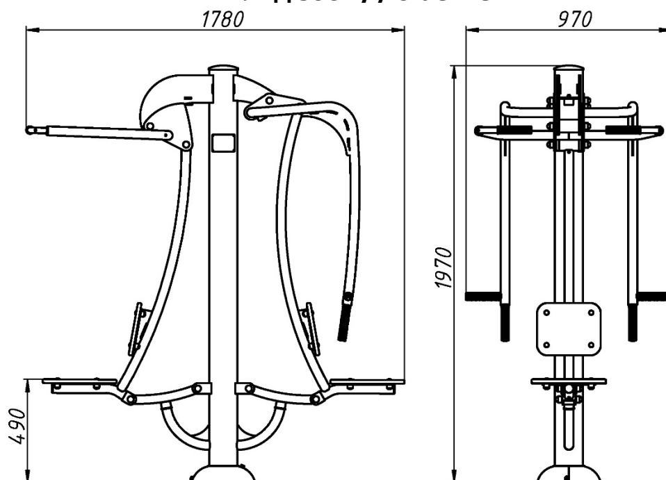
Вигляд збоку / Side view
