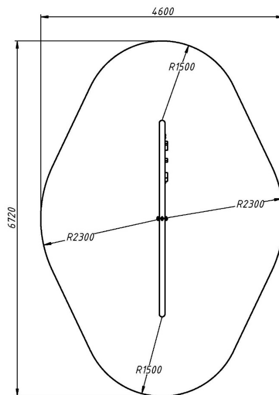
Вигляд зверху, враховуючи зону безпеки / Top view, including the safety zone
