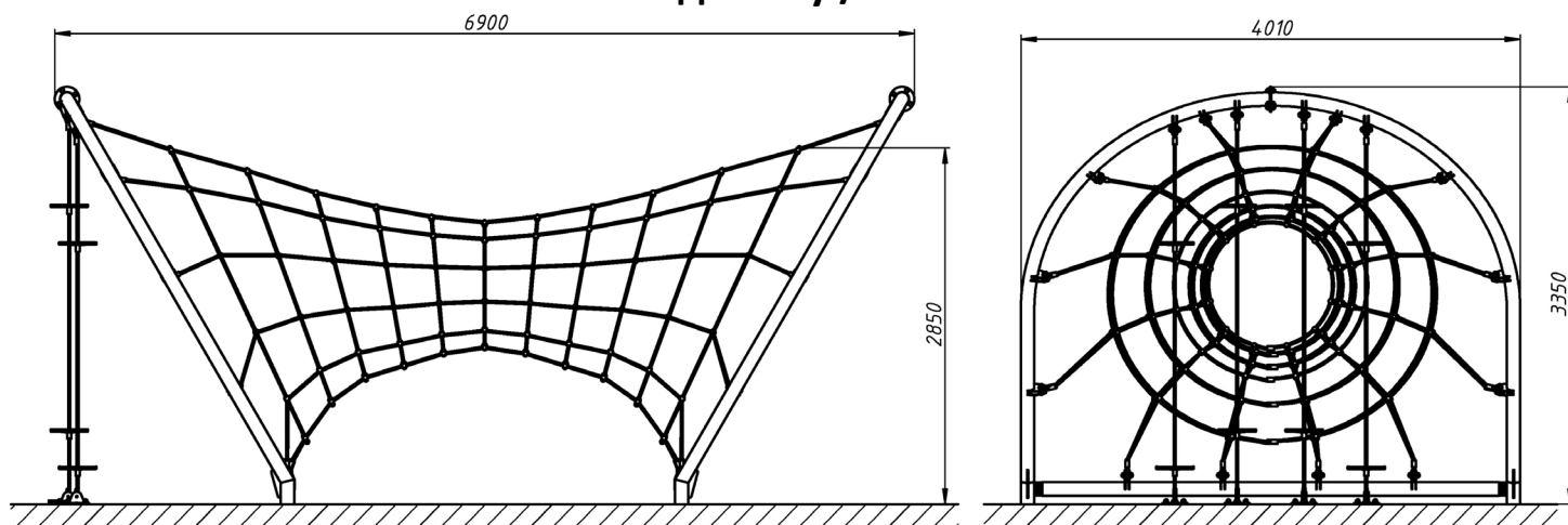
Вигляд збоку / Side view
