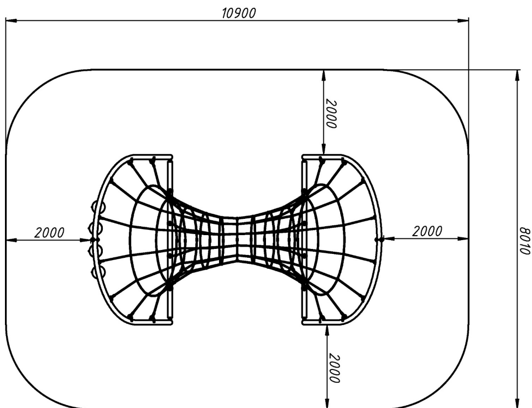
Вигляд зверху, враховуючи зону безпеки / Top view, including the safety zone
